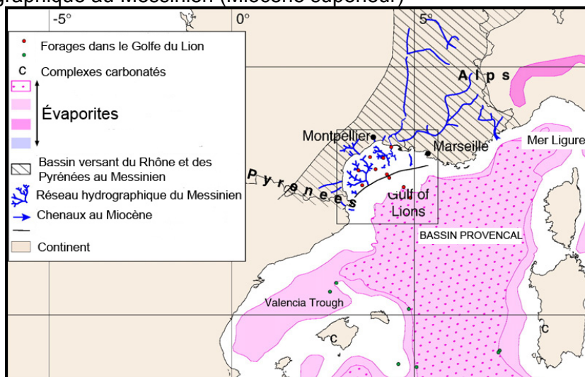
Document 1d : carte de localisation des séries évaporitiques en Méditerranée occidentale et réseau hydrographique au Messinien (Miocène supérieur)
